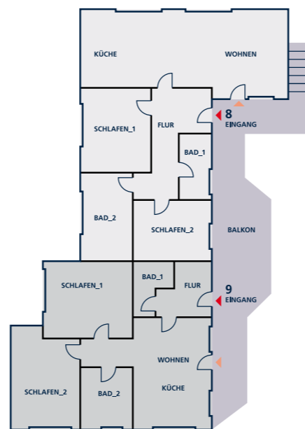
Grundriss: Wohnungen 8+9
